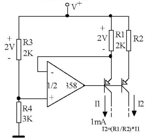
固定电流源
